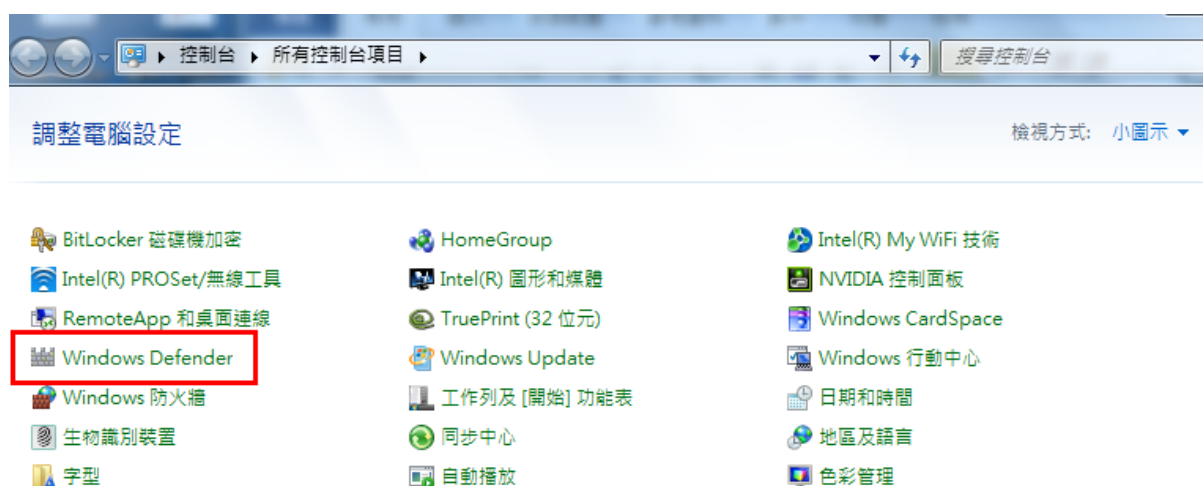
圖8 啟動 Defender
